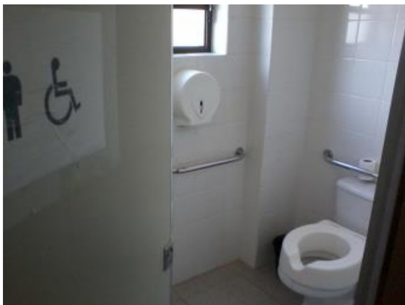
Figura III – Banheiro adaptado para cadeirantes.
